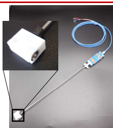
耐酸性インライン温度センサ
